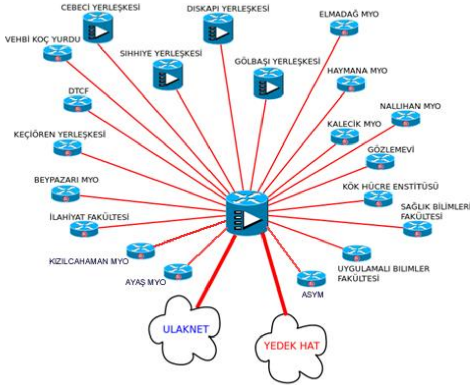
Şekil 3: Ankara Üniversitesinin Ağ Topolojisi
