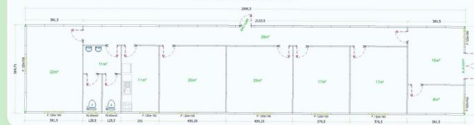
169m 2 PREFABRİK BİNA PLANI
