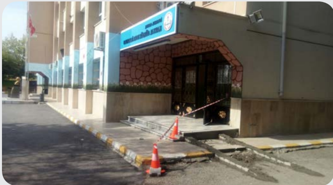
Gülbüz Bora İlköğretim Okulu Engelli Rampası Yapımı
