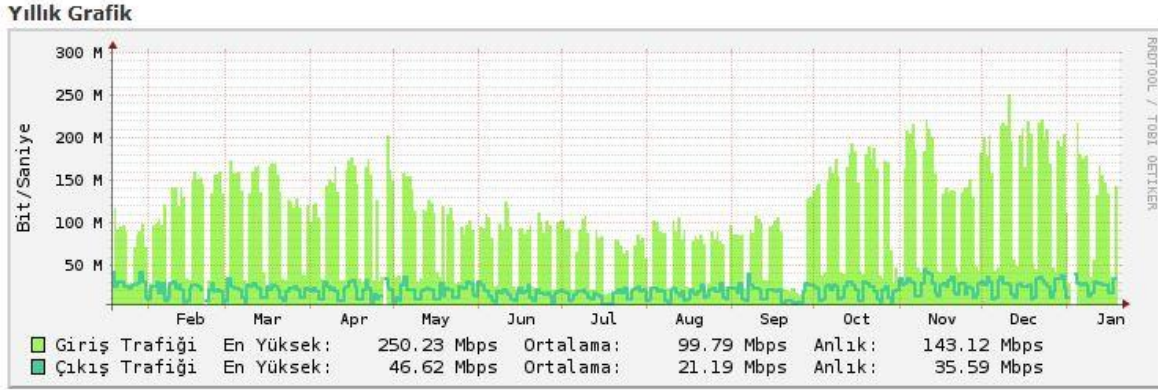
Şekil 1. Balıkesir Üniversitesi ULAKNET Grafiği (2015)
