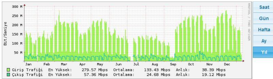
Şekil 2. Balıkesir Üniversitesi ULAKNET Grafiği (2016)
