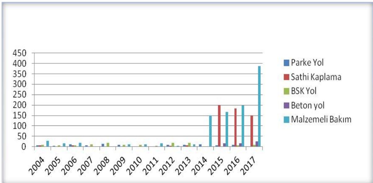
Çarşamba Belediyesi 2004-2017 Yılları Arası Yol Çalışmaları Grafiği (km/yıl)
