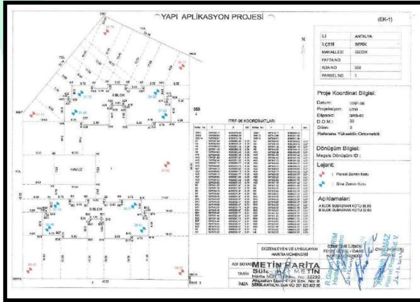
Şekil 15: Yapı Aplikasyon Krokisi
