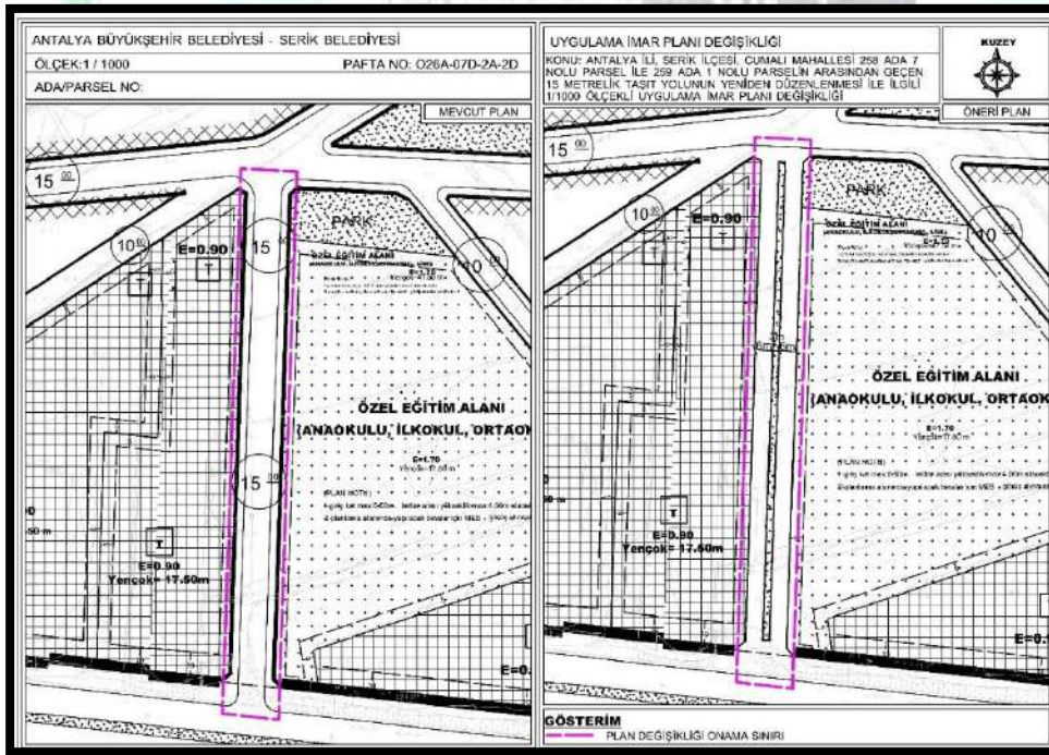
Şekil 31 : Antalya İli, Serik İlçesi, Cumalı Mahallesi 258 ada 7 parsel 1/1000 Ölçekli Uygulama İmar Planı Değişikliği
