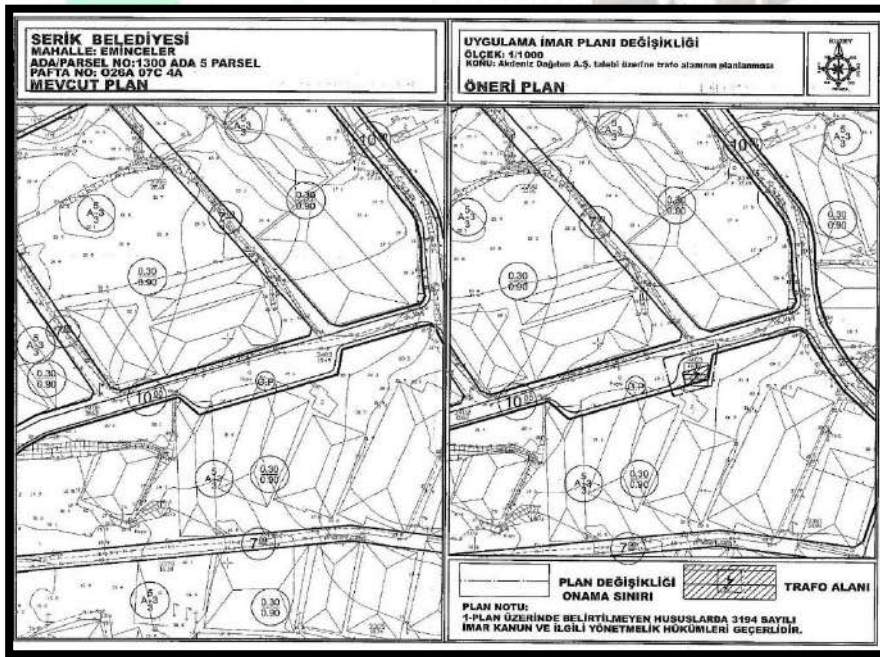
Şekil 44 : Antalya İli, Serik İlçesi, Eminceler Mahallesi 1300 Ada 5 Parsel Kuzeyinde Bulunan Otopark Cebine Trafo Konulması 1/1000 Ölçekli Uygulama İmar Planı Değişikliği
