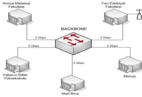
Davutpaşa Kampüsü Network Altyapısı
