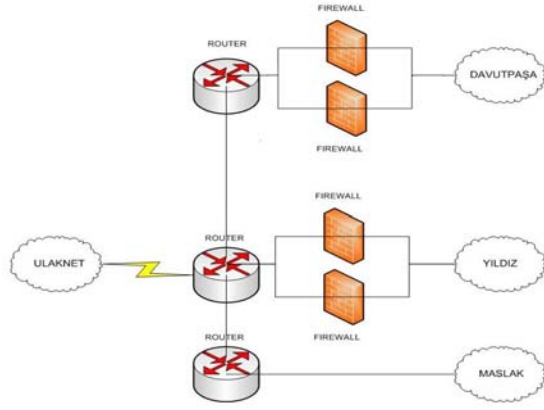
Kampüslerimiz Arası Network Altyapısı
