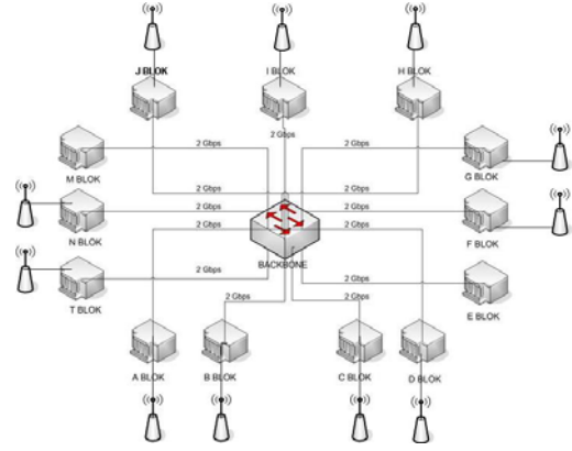
Yıldız Merkez Kampüsü Network Altyapısı
