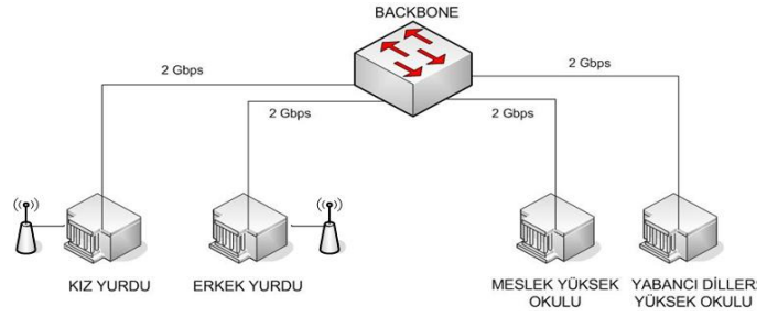
Maslak Kampüsü Network Altyapısı
