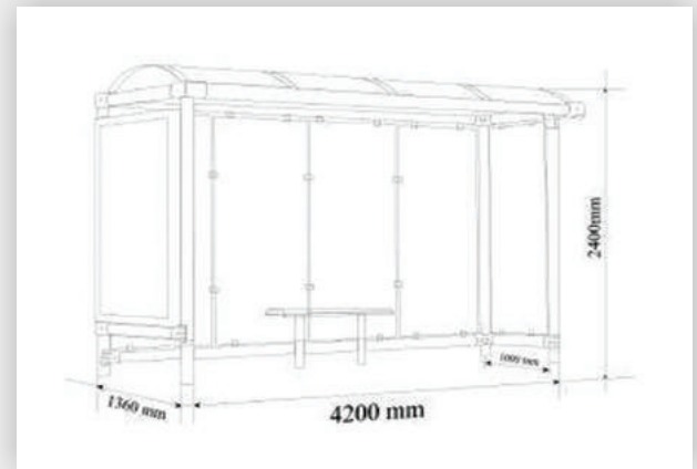
Hazırlanan Proje
