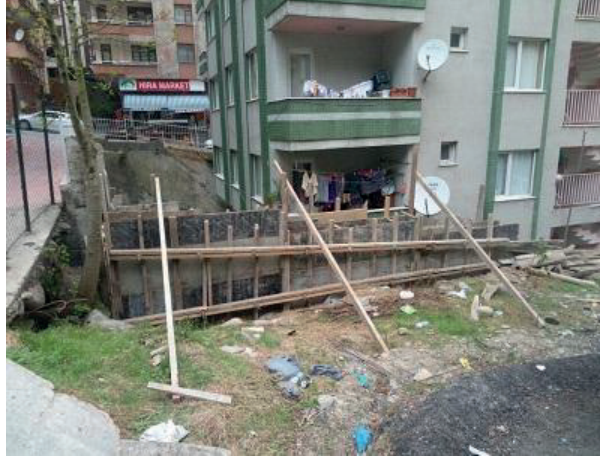
1 Nolu Dere Sokak'ta perde duvar ve yol betonlama çalışmaları
