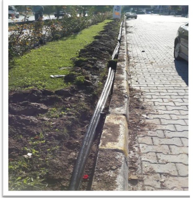
Görüntü 46. Gaziosmanpaşa Caddesi Kahve Durağı Önü Yeşil Alanı Otomatik Sulama Sistemi Kurulum Çalışmaları
