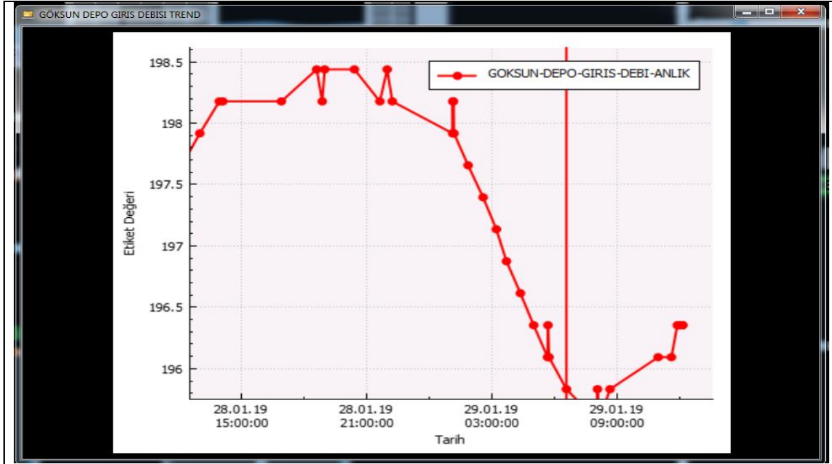
Şekil 19. Göksun Deposu giriş debisinin geçmiş verilerinin izlenmesi
