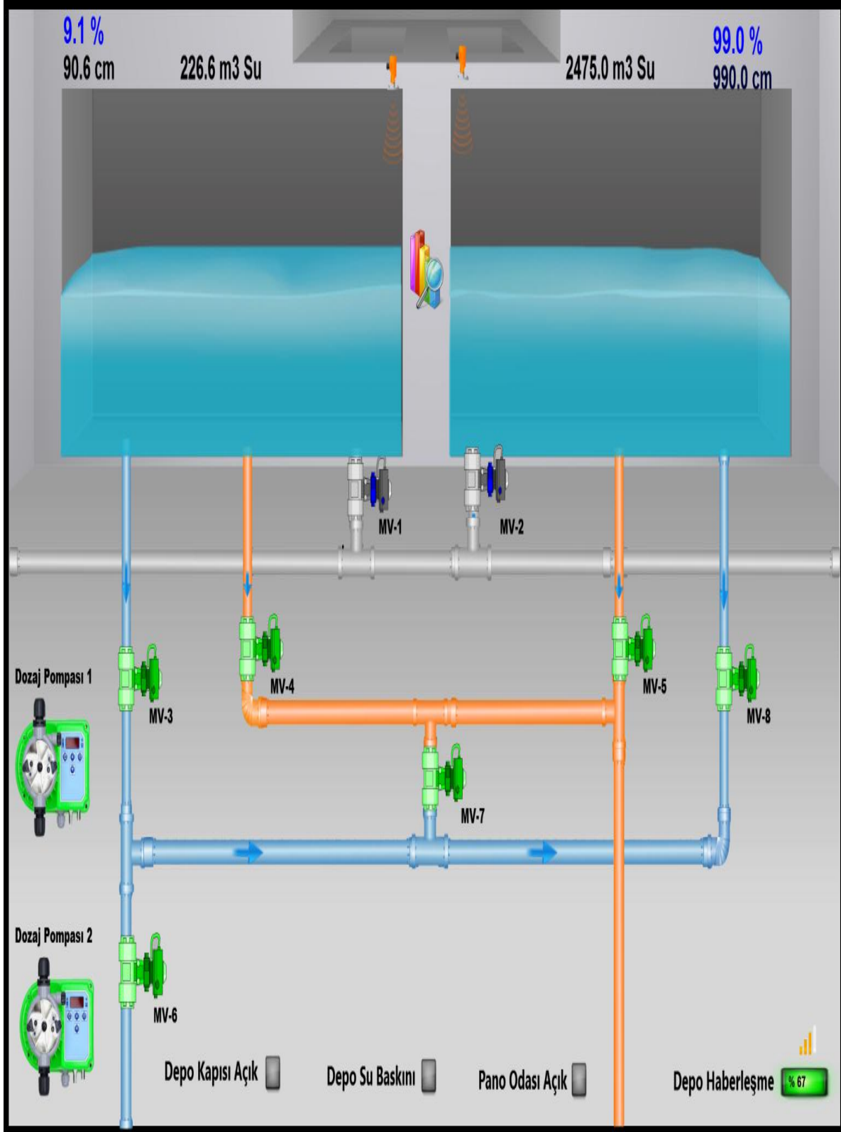
Şekil 21. Gökşun Deposu manevra odasının KASKİ SCADA ekranında izlenmesi
