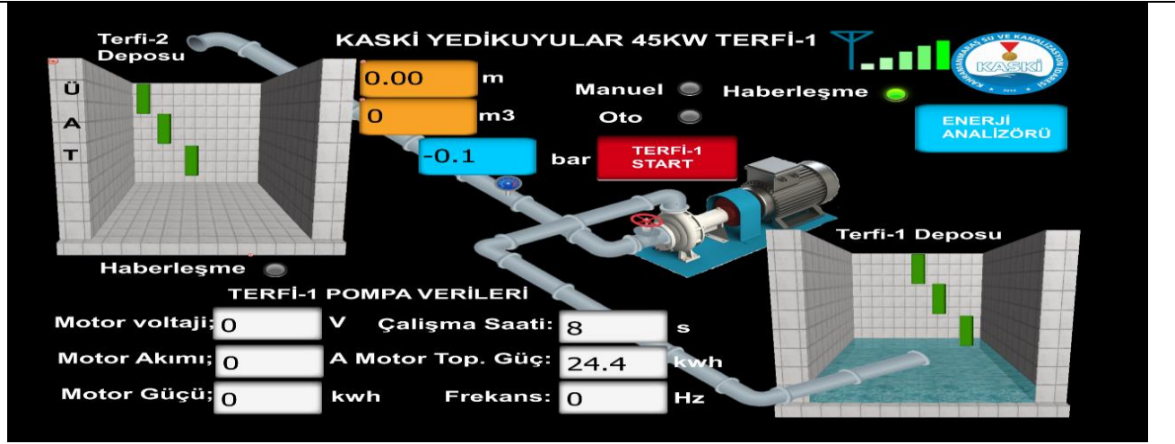
Şekil 17. Yedikuyular içmesuyu şebekesinin 1. Terfi noktasının KASKİ SCADA ekranında izlenmesi
