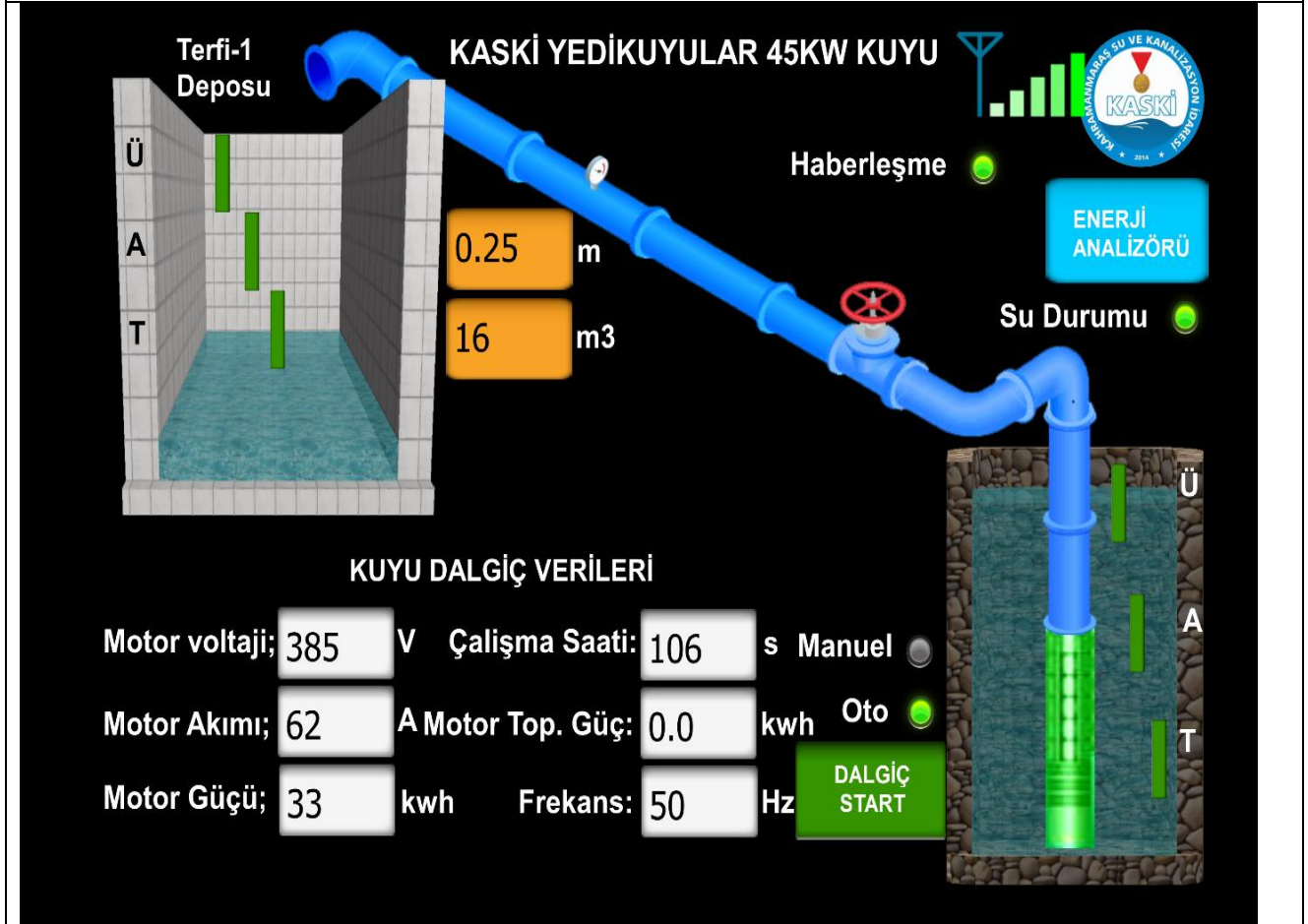
Şekil 16. Yedikuyular içmesuyu şebekesinin kuyu sondajının KASKİ SCADA ekranında izlenmesi
