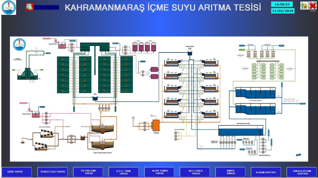
Şekil 14. Kullanılan CIMON SCADA programı ana ekranı
