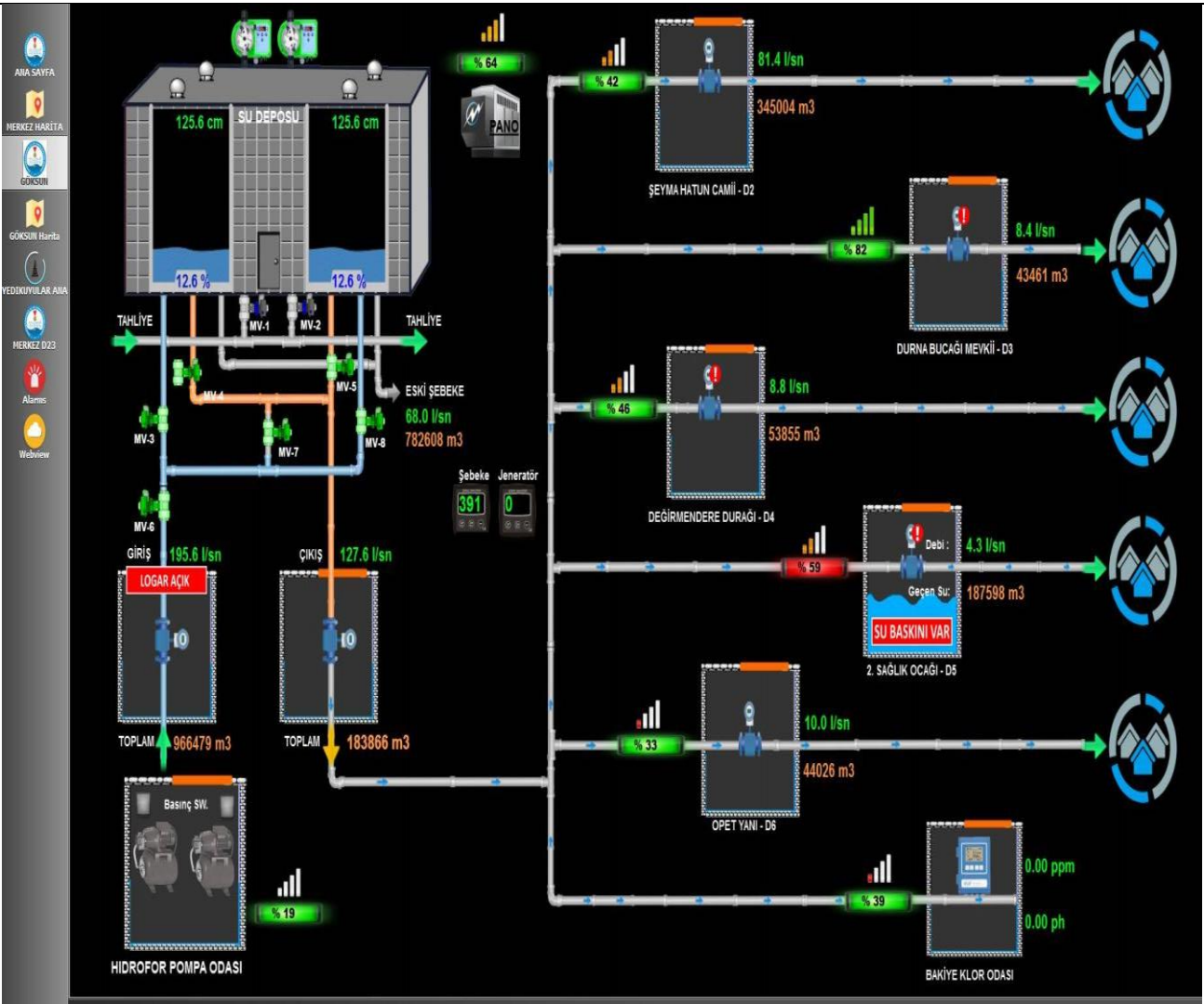
Şekil 17. Yedikuyular içmesuyu şebekesinin 1. Terfi noktasının KASKİ SCADA ekranında izlenmesi
