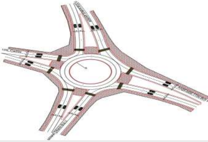
Karaköprü Mimar Sinan Kavşak Düzenleme Çalışması
