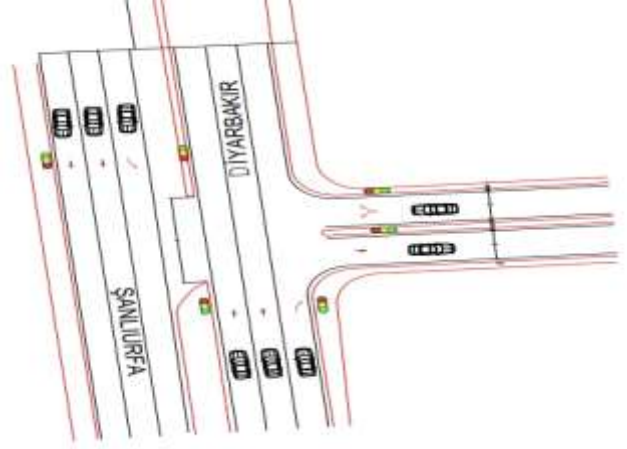
Karaköprü Metrolife Hastane Kavşak Düzenleme Çalışması
