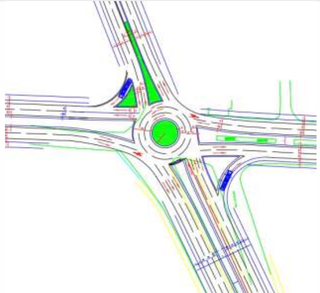
Karaköprü Maşuk Kavşak Düzenleme Çalışması
