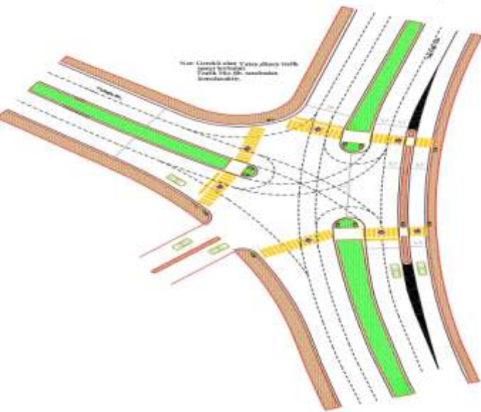
Karaköprü Yeşiloğlu Bulvarı Kavşak Düzenleme Çalışması
