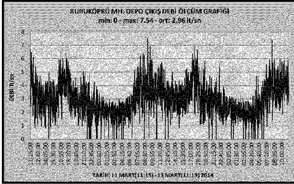
ÖRNEK DEBİ GRAFİĞİ
