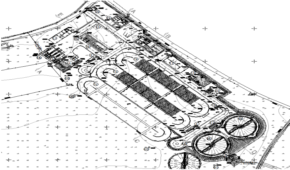
Atıksu Arıtma Tesisi Yerleşim Planı
