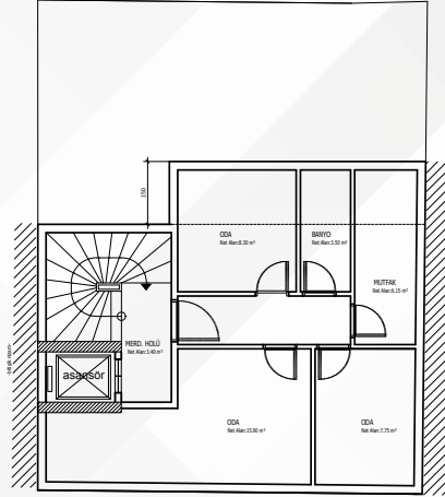
1.2. ve 3. NORMAL KAT PLANI NORMAL KAT ALANI: 68.00 m 2 ÖNERİ-1
