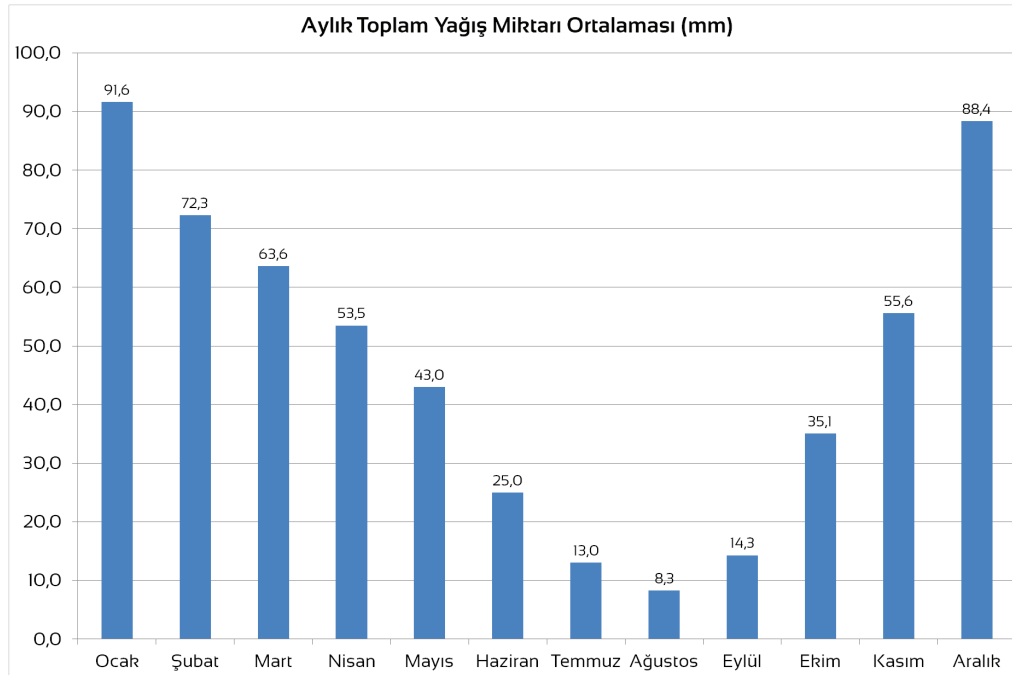
Grafik 1 – 2017 Aylık Toplam Yağış Miktarı Ortalaması (kg/m 2 )
