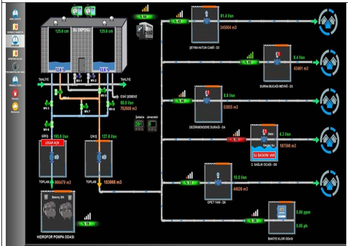
Göksun İlçe Merkezi içme suyu şebekesinin KASKİ SCADA ekranında izlenmesi
