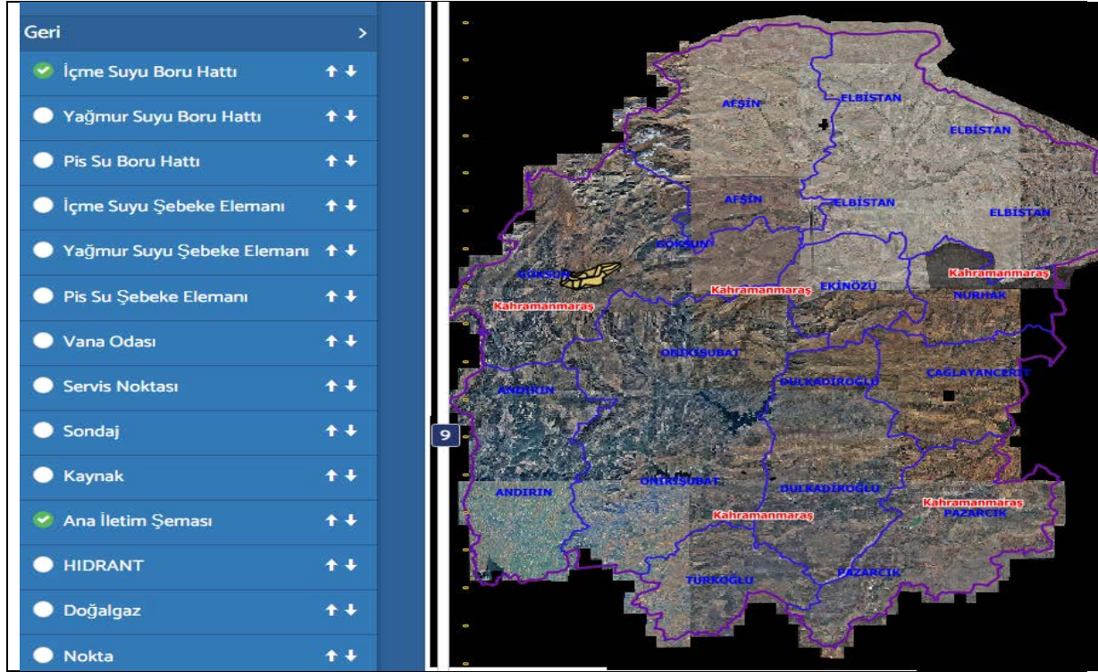
Şekil 1. CBS Portal
