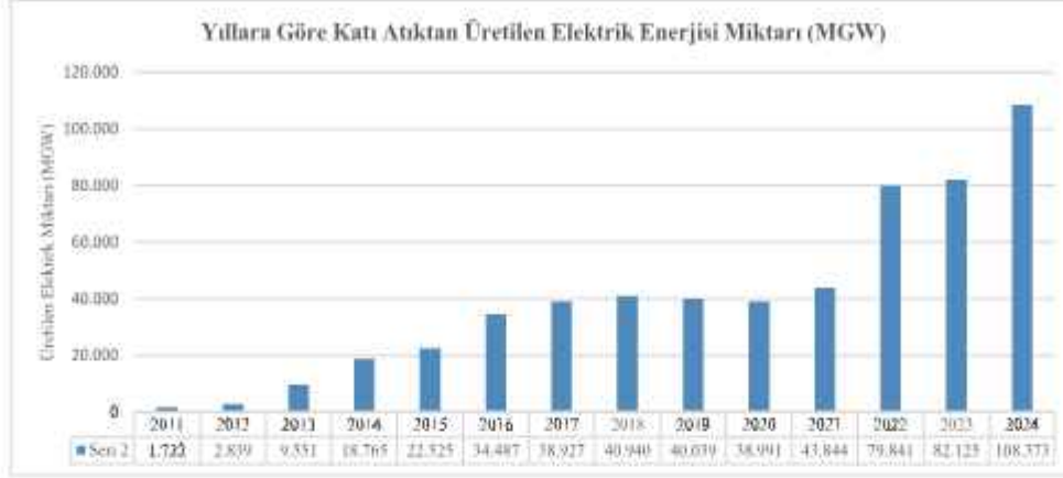
Grafik 5 Yıllara Göre Merkez Saha Katı Atıktan Üretilen Elektrik Enerjisi Miktarı (MGW)
