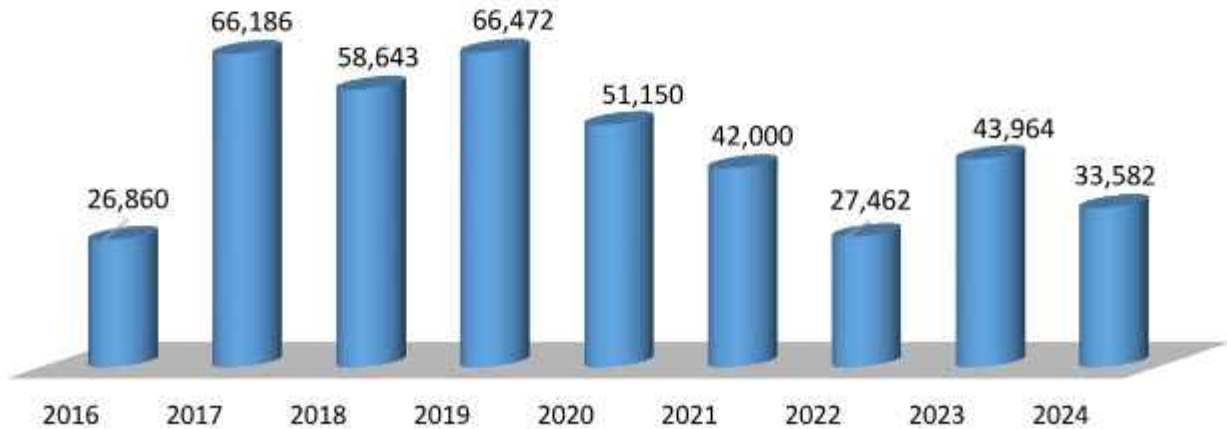
Grafik 40 Yıllara Göre İmalatı Yapılan İçme Suyu Hattı (Metre)
