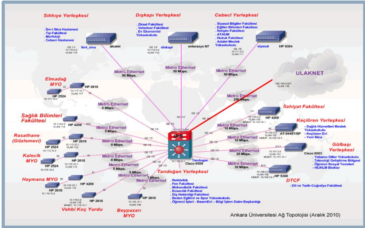
Şekil-3 Ağ Topolojisi
