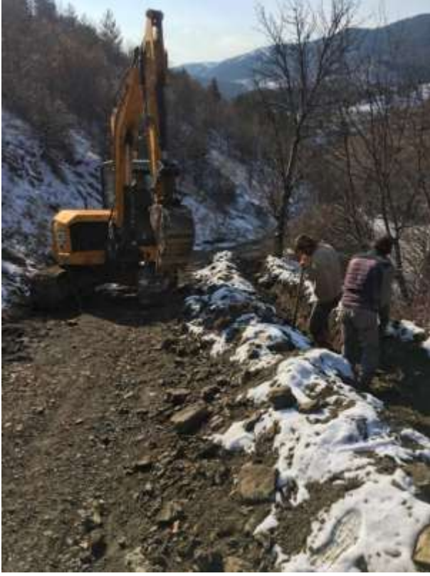
Merkez Çaltılı Köyü Limit İçmesuyu İnşaatı
