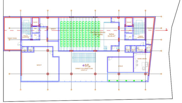
-2. BODRUM KAT PLANI Ö: 1/50
