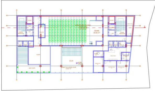
-1. BODRUM KAT PLANI Ö: 1/50
