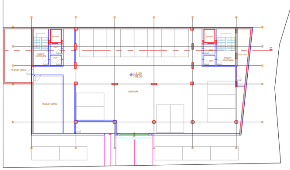
-3. BODRUM KAT PLANI Ö: 1/50
