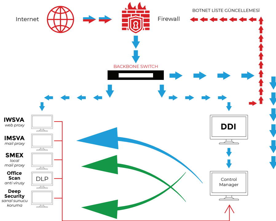
Şekil : Güvenlik Yazılımları Topolojisi
