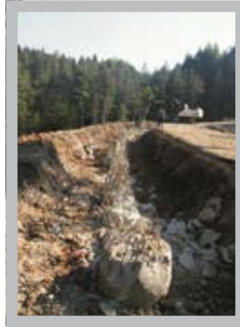
Çınardüzü Köyü Heyelan Önüne Taş Duvar Yapım İşİ
