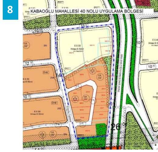
PLAN GÖRÜNÜMÜ
