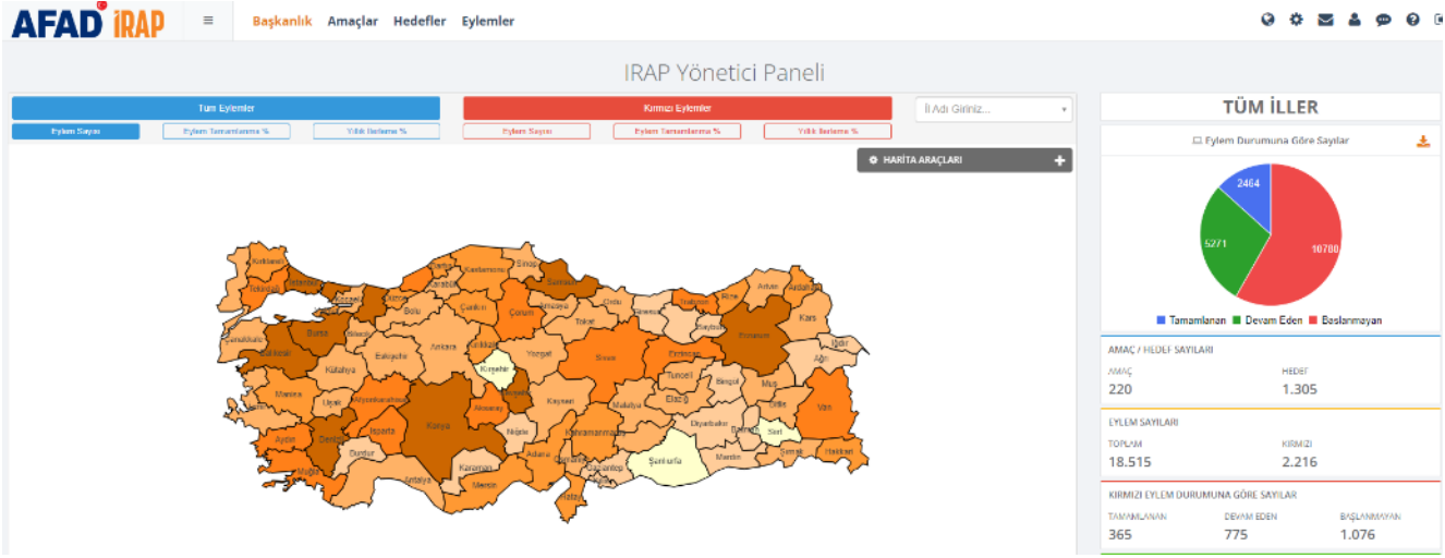
Şekil 13 - İRAP Yazılımı
