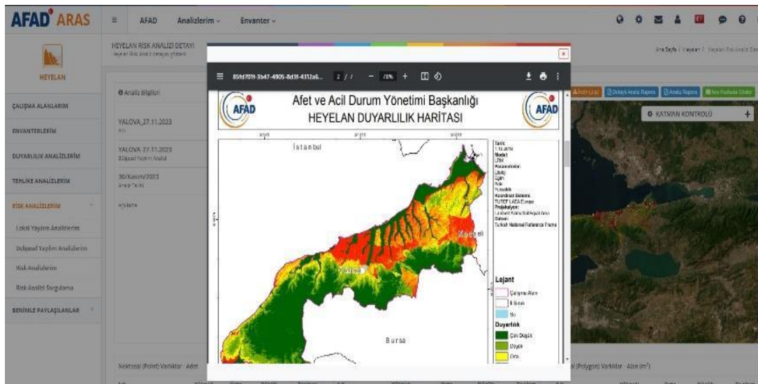
Şekil 14 - Heyelan Risk Analizi
