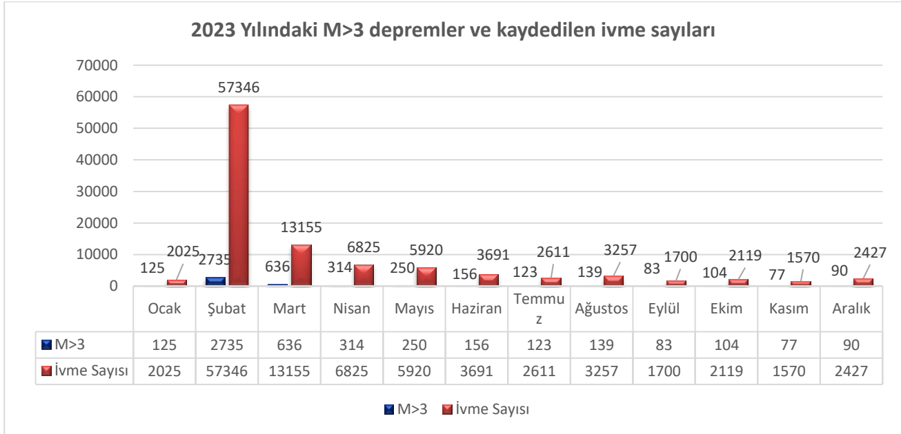
Şekil 17 - 2023 Yılı M>3 Deprem ve İvme Sayıları Grafiği
