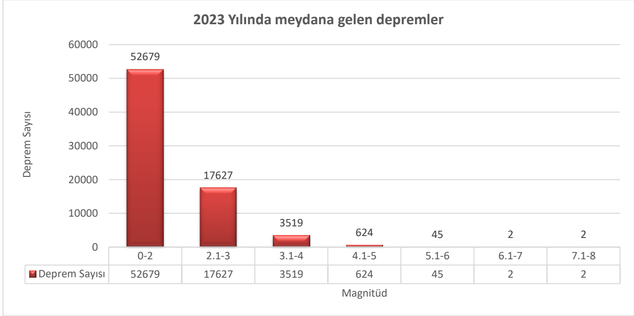
Şekil 16 - 2023 Yılı Deprem Sayısı-Büyüklüğü Grafiği
