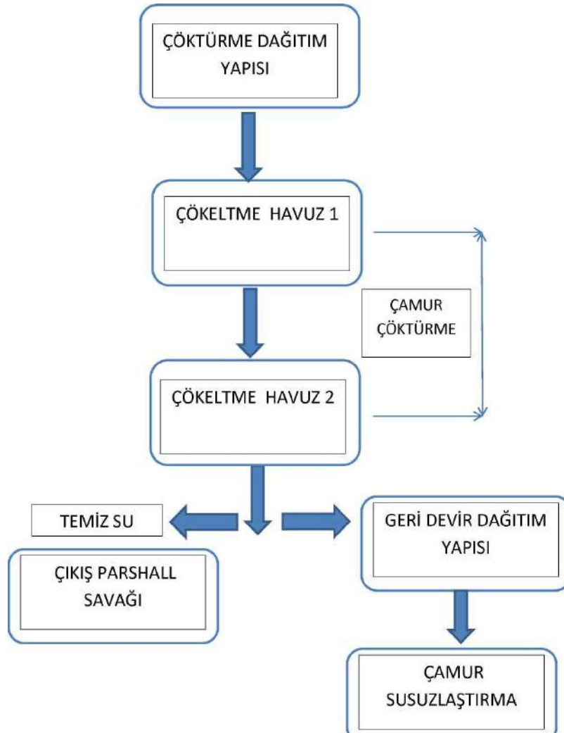
Şekil 3.5 Çöktürme Havuzu Ünitesi İş Akım Şeması
