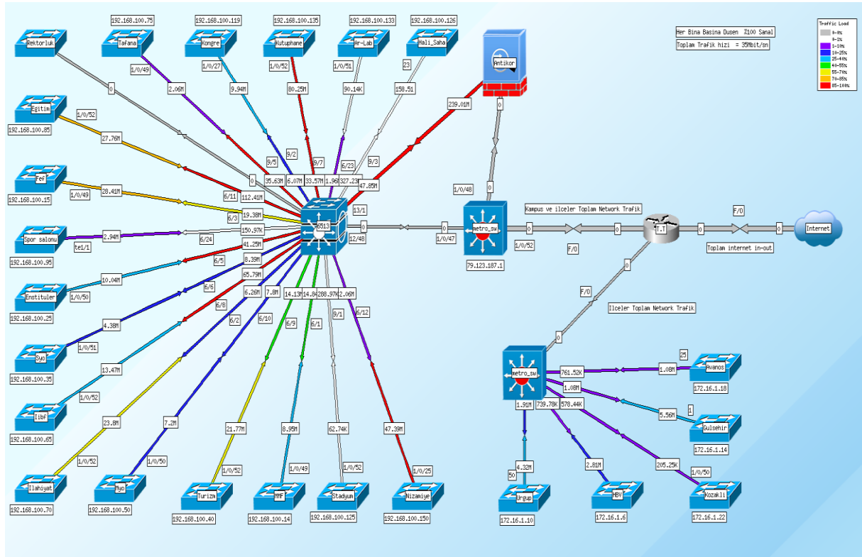
Şekil 2: Neü/Net Topoloji
