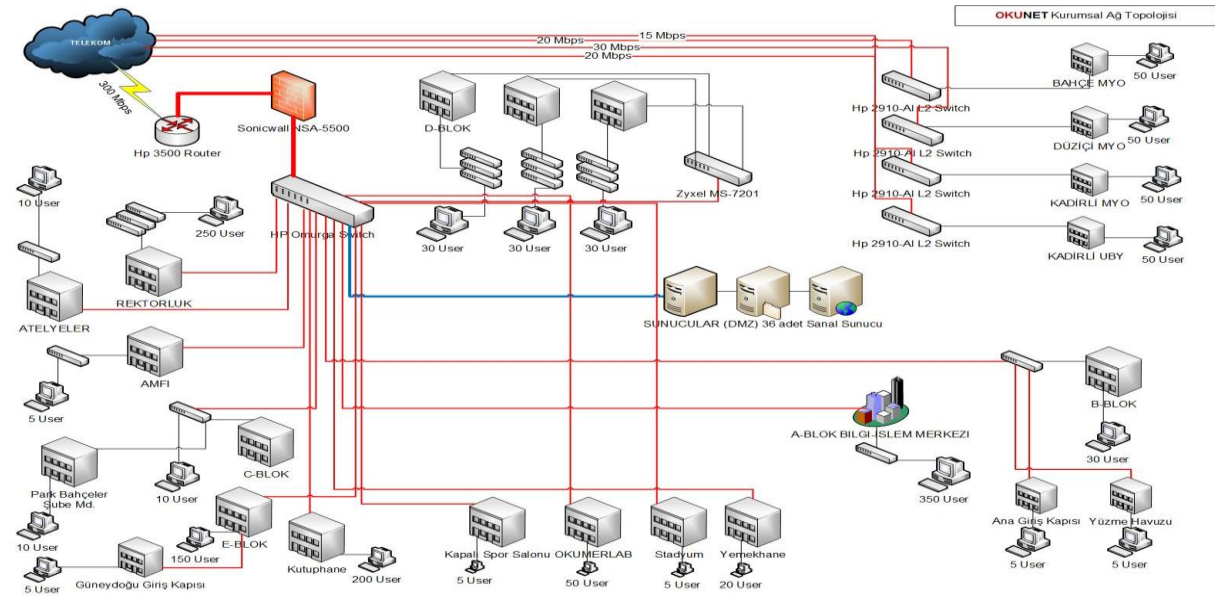
Şekil 2: OKÜ Ağ Planı
