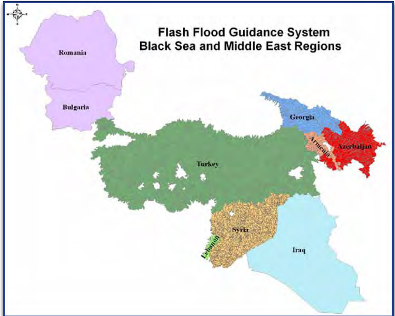
Şekil-45: Karadeniz ve Ortadoğu Bölgesel Ani Taşkın Erken Uyarı Merkezine dahil ülkeler
