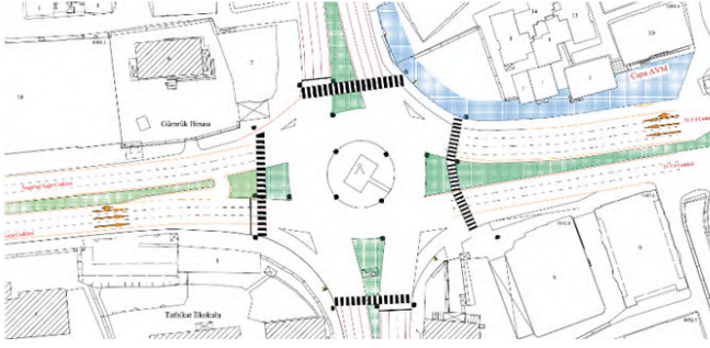
Yakutiye İlçesi Gez Sinyalizasyonlu Kavşak Projesi
