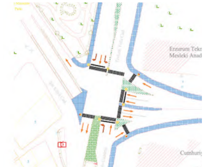
Yakutiye İlçesi Tortum Yolu - Şıh Köyü Caddesi Sinyalizasyonlu Kavşak Projesi
