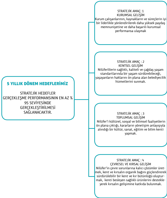
Şekil 2.1. Stratejik Amaçlarımız
