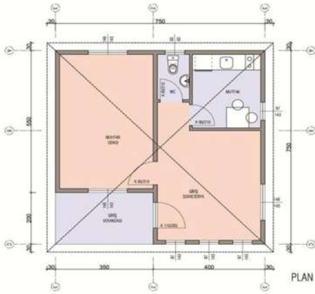
Yenimahalle Muhtarlık Binası Mimari Çizimleri
