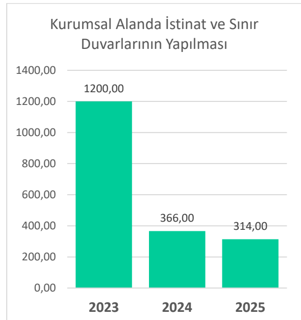
Kurumsal Alanda İstinat ve Sınır Duvarlarının Yapılması Tablosu (m²)
