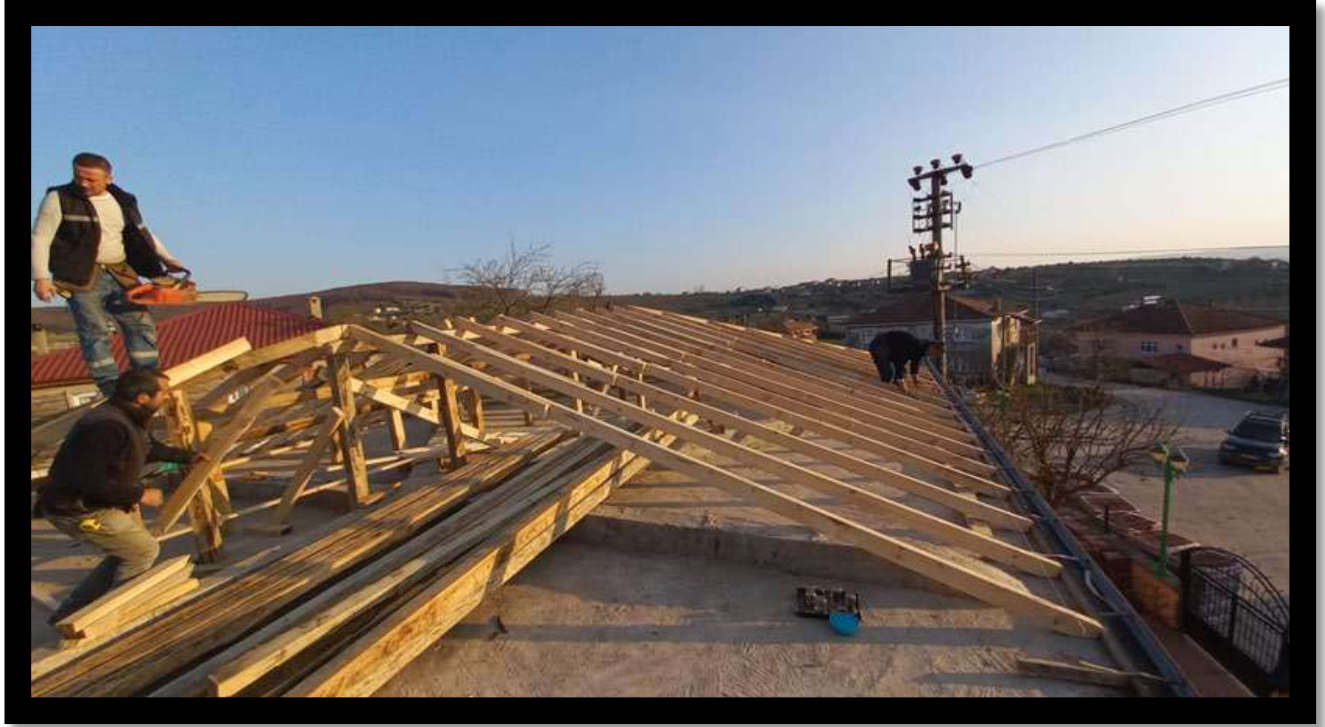
Avdan Mahallesi Merkez Camii Çatı İmalat Çalışması
