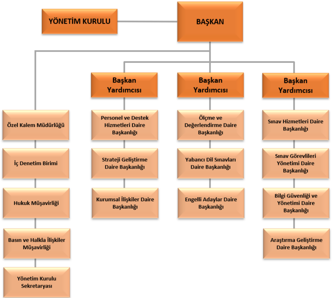
Şekil 1- Teşkilat şeması
