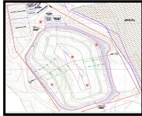
Gökçeğöz Düzenli Depolama ve Bertaraf Tesisi Vaziyet Planı
