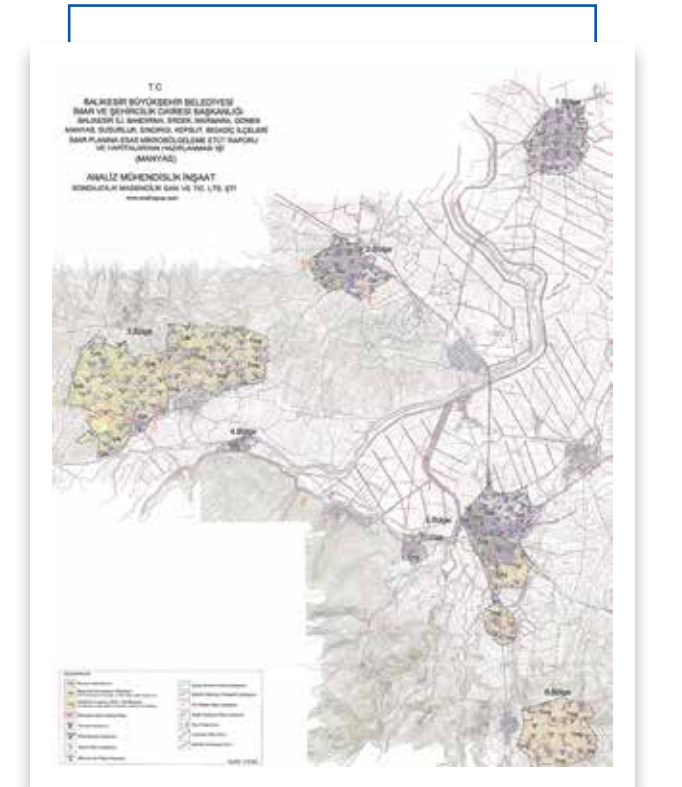
Manyas Sondajlar ve Jeoloji Haritası
