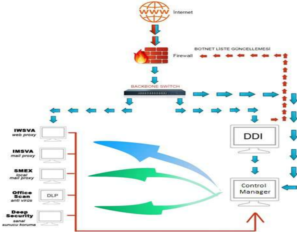
Şekil 2: Güvenlik Yazılımları Topolojisi
