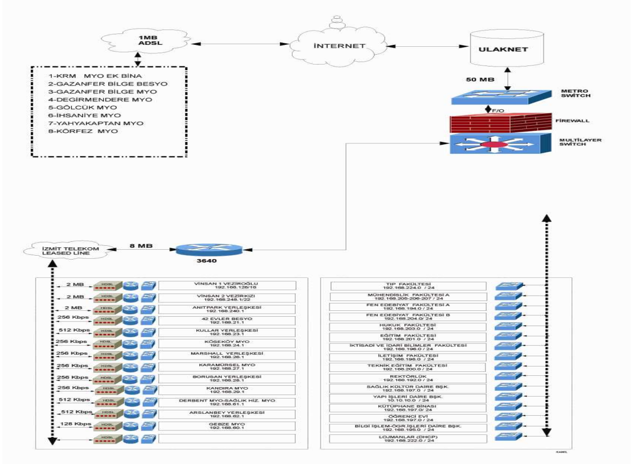
Şekil 2- Umuttepe Yerleşkesi Fiber Optik Ağ Şeması
