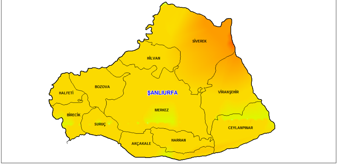
Şekil 1 http://www.naturelenerji.com.tr/Gunes_Enerjisi_Potansiyeli_Atlasi_GES.aspx?SehirID=63
